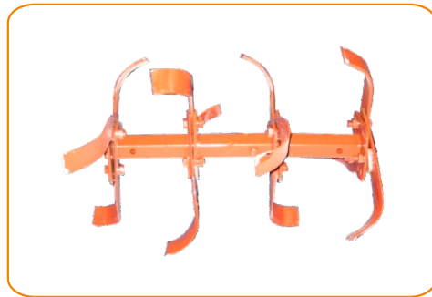
刀具名称 三片四组旱地刀
