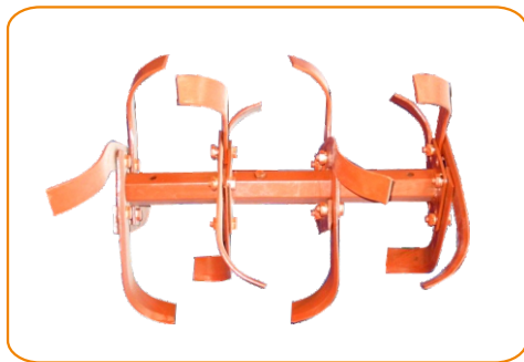
刀具名称 四组四片旱地刀
